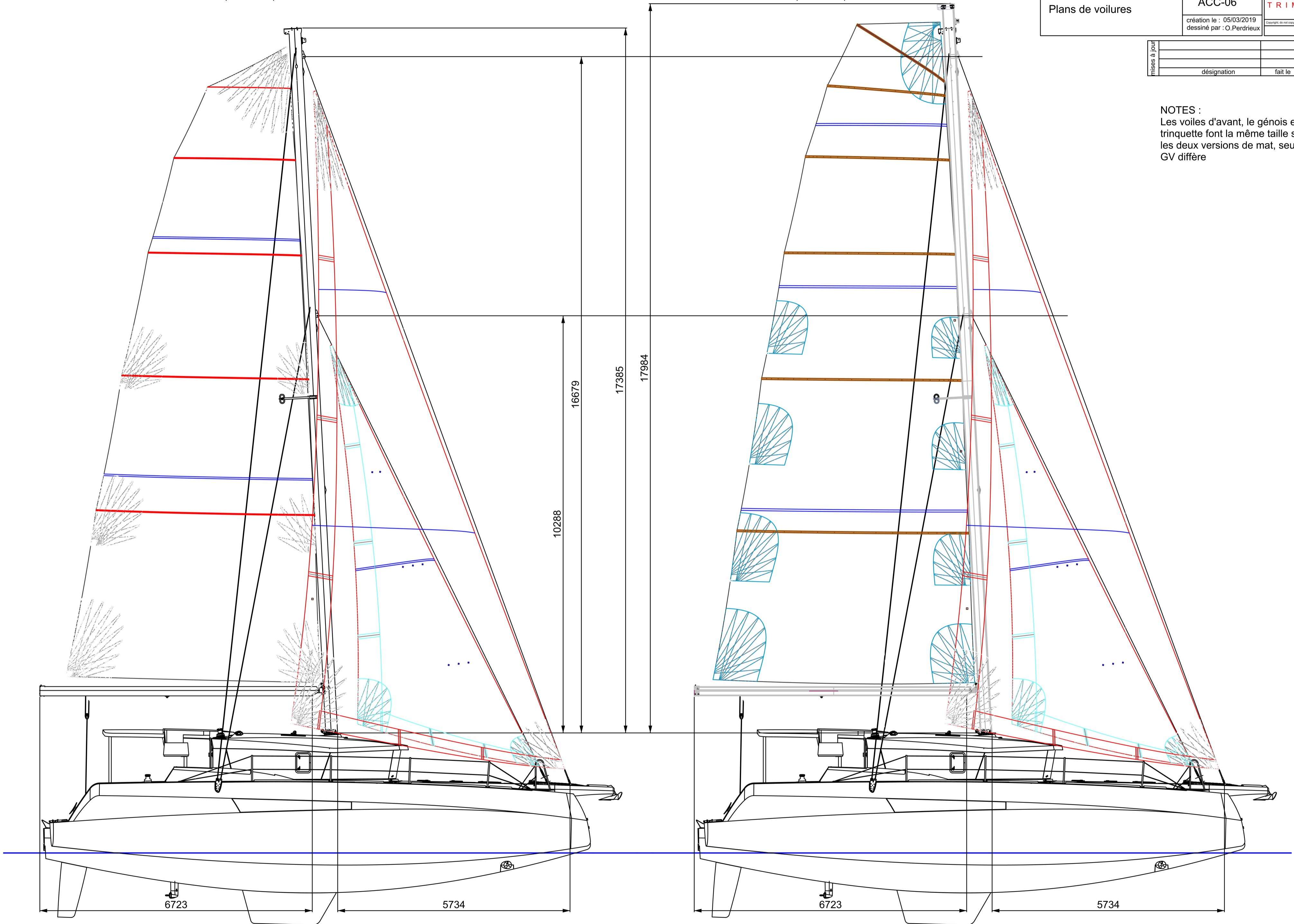
Plan de voile du mat alu (GV à 2 ris)
