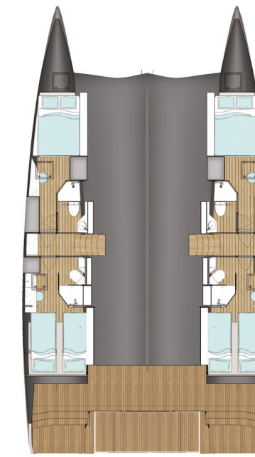
5 cabins / 8 pax 5 cabines / 8 personnes
