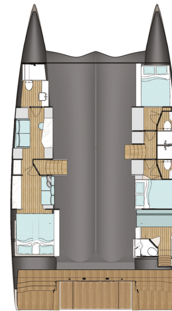
4 cabins / 6 + 2 pax 4 cabines / 6 + 2 personnes
