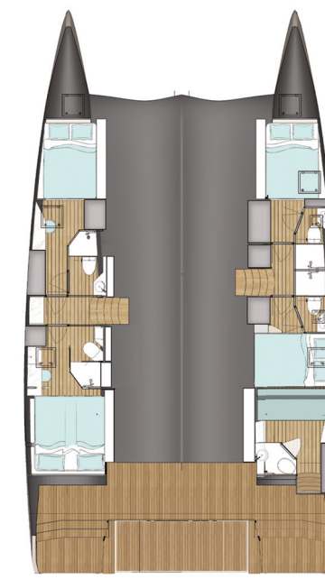
5 cabins / 8 + 2 pax 5 cabines / 8 + 2 personnes
